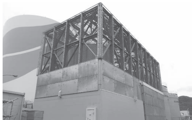
↑竜巻対策として飛来物によるタンクの損傷を防ぐ防護ネット
