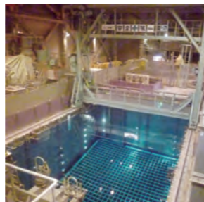
↑使用済燃料プール
