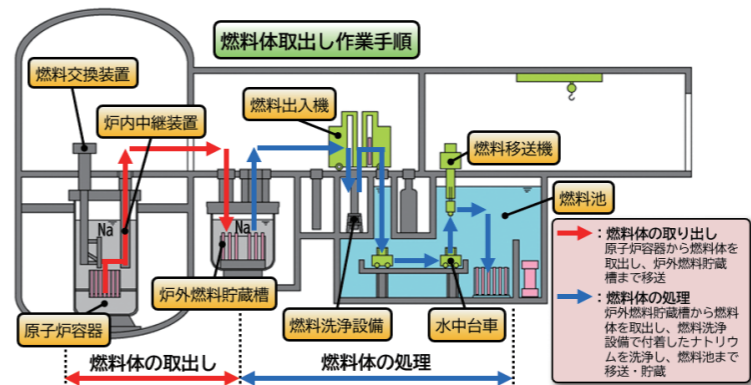
↑ 燃料体取り出しの概要
