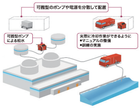
↑ 代替設備による原子炉冷却のイメージ
